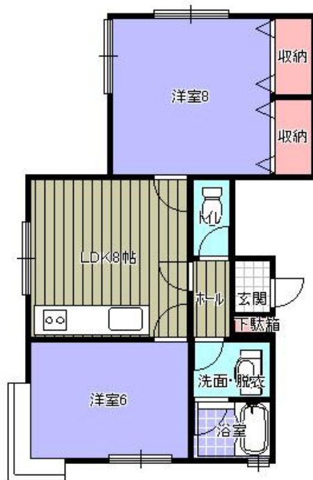
2階 平面図
