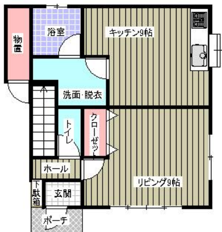
1階 平面図
