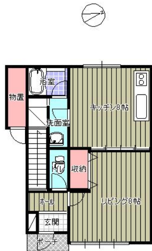
1階 平面図
