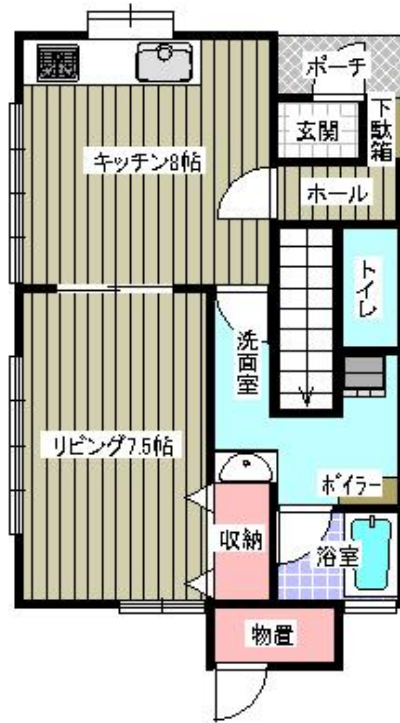
1階 平面図
